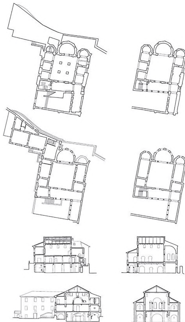
Рис. 7. Резиденция епископа в Порче середины VI в., Хорватия. Планы. Слева: до реставрации; справа: после реставрации. Продольные и поперечные разрезы. По П. Шевалье и И. Матейчичу [17, fig. 3]
