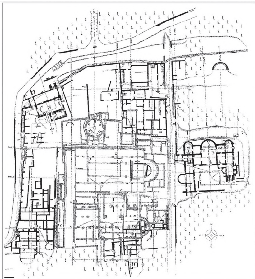
Рис. 4. Епископский квартал в Салоне IV–VI вв., Хорватия. План по В. Герберу [22, fig. 2]
