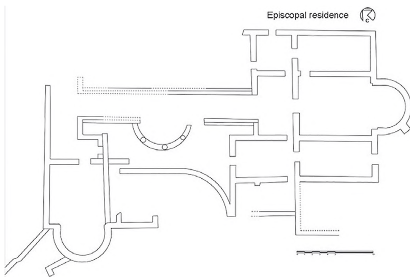
Рис. 2. «Епископская резиденция» в Стоби IV–VI вв., Северная Македония. План [32, fig. 77b]
