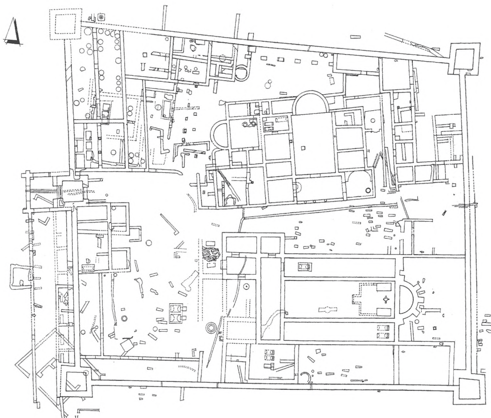
Рис. 9. Епископский комплекс в Лулудиее к. V — сер. VI вв., Греция. План по Э. Марки, Ц. Булосу [45, fig. 4]
