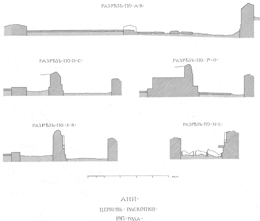
Рис. 2. А. П. Удаленков. Ани. Разрезы раскопанной в 1917 г. церкви. РО НА ИИМК РАН. Р-І. Оп. І. Д. 141. Инв. 951
