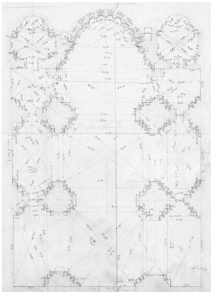
Рис. 4. А. П. Удаленков. Ани. Обмеры собора. Внутренний обход. 1917 г. РО НА ИИМК РАН. Р-1. Оп. 1. Д. 141. Инв. 971
