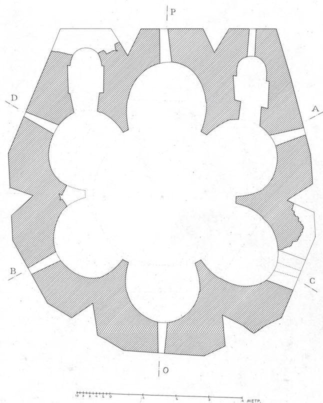
Рис. 11. А. П. Удаленков. Ани. План монастырской церкви Абуханма в Вышгороде. РО НА ИИМК РАН. Р-І. Оп. 1. Д. 141. Инв. 956
