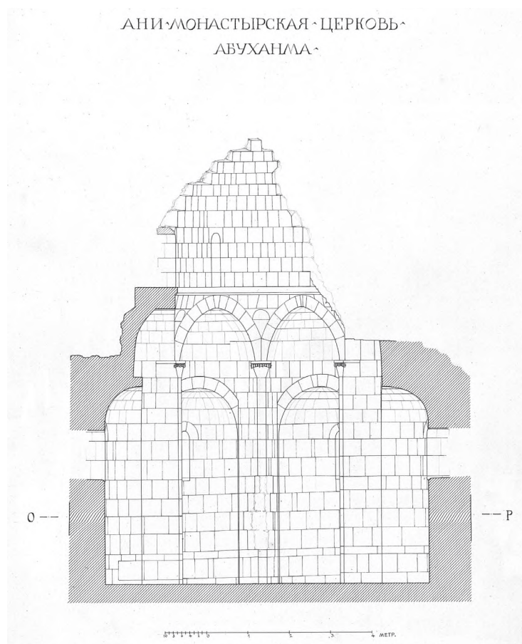
Рис. 12. А. П. Удаленков. Ани. Разрез монастырской церкви Абуханма в Вышгороде. РО НА ИИМК РАН. Р-І. Оп. 1. Д. 141. Инв. 966
